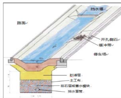
场地与道路——草沟
